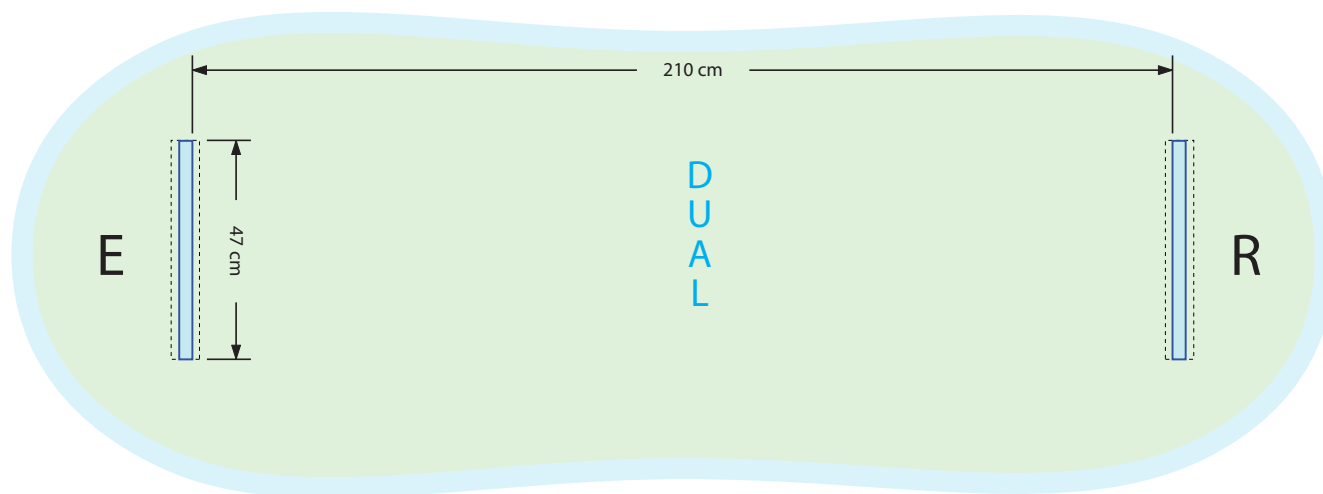
Portique classique émetteur récepteur AM47 , en coupant le récepteur du transceiver en vert : la zone de couverture utile, en bleu la zone incertaine. Très peu de couverture arrière.
