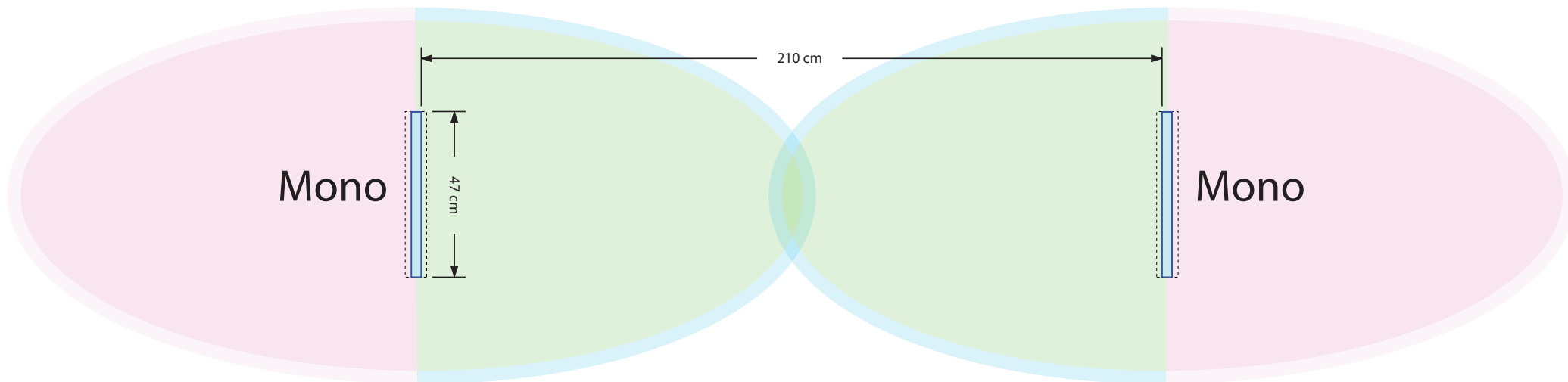
Double MONO ANTENNE AM47 (portée 105 cm avec Ultrastrip 3+1) en vert : la zone de couverture utile, en bleu la zone incertaine, en rose la couverture arrière
